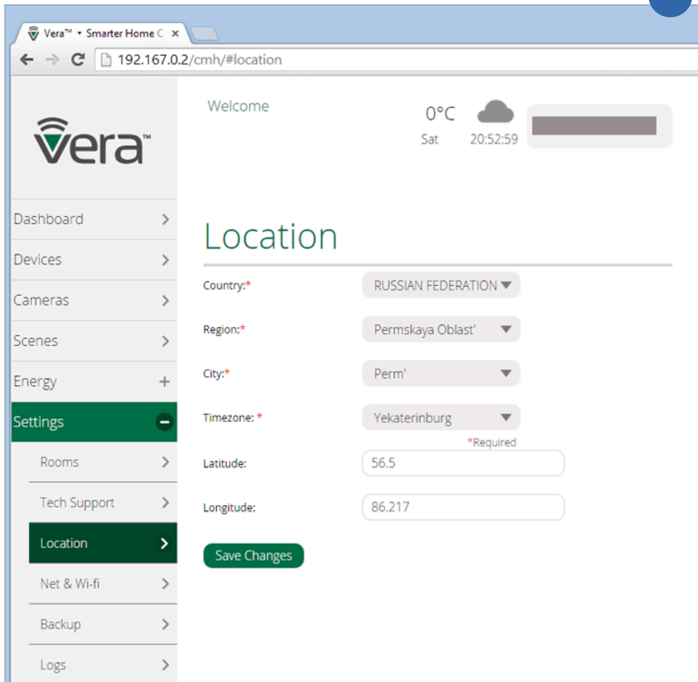
Рис. 16. Настройки местоположения
